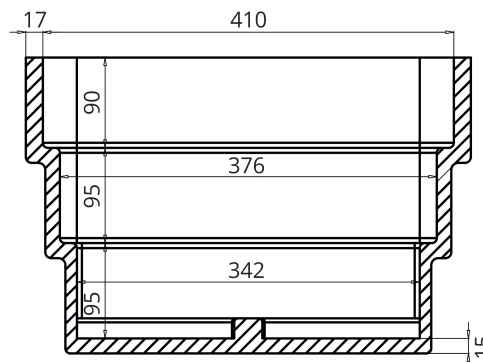
SECCIÓN A-A
