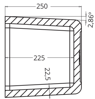
SECCIÓN A-A
