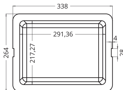
PLANTA SUPERIOR
