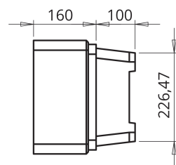
ALZADO LATERAL
