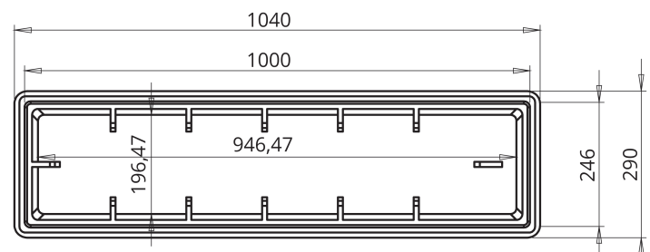
PLANTA SUPERIOR
