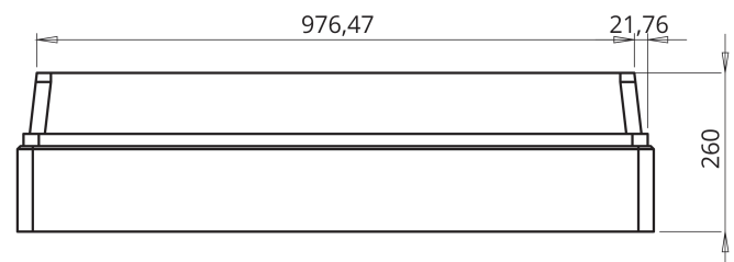
ALZADO FRONTAL
