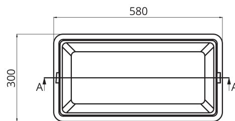
PLANTA SUPERIOR
