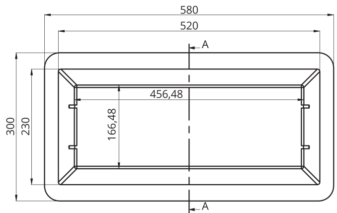
PLANTA SUPERIOR
