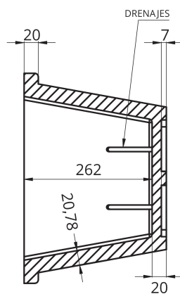
SECCION A-A
