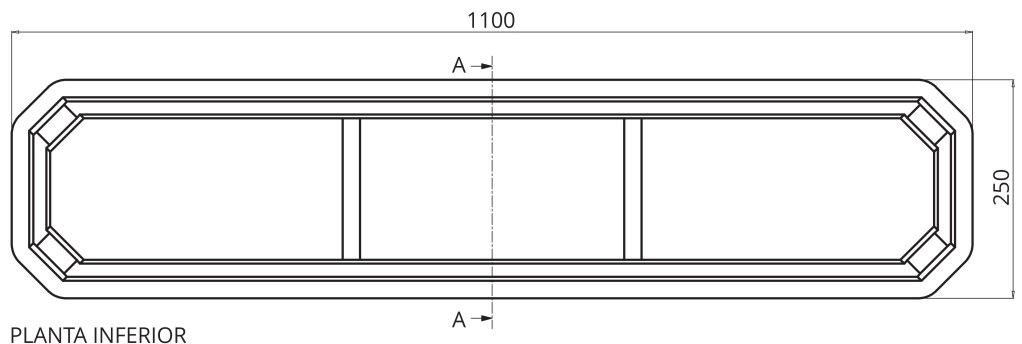
PLANTA INFERIOR
