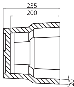
SECCION A-A
